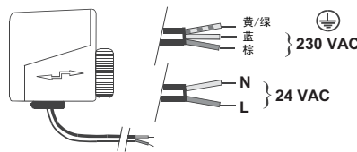
接线图
