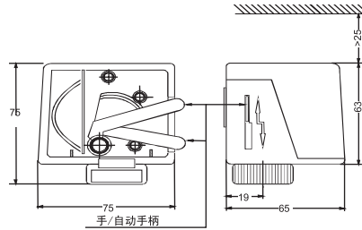
尺寸 (mm)
